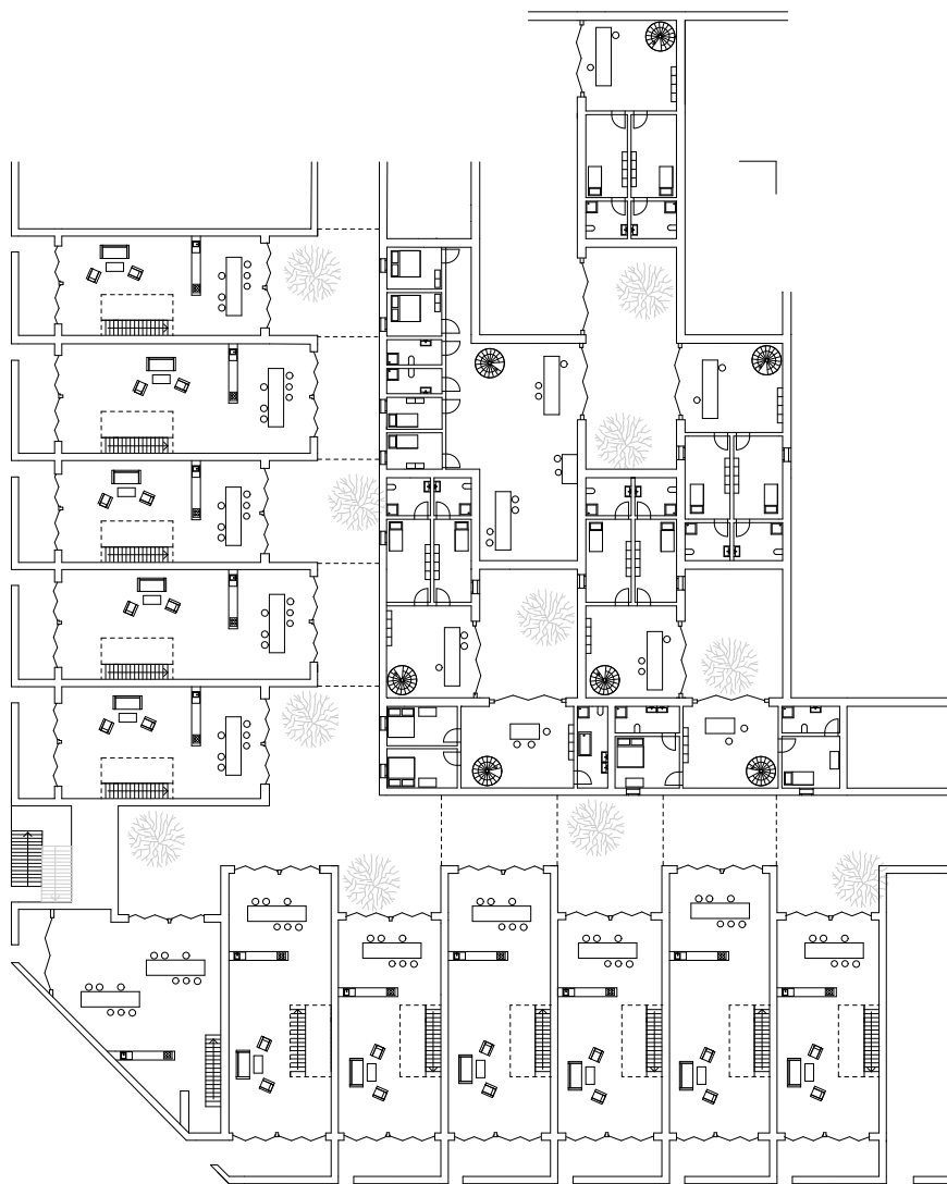
Grundriss EG 1:200
