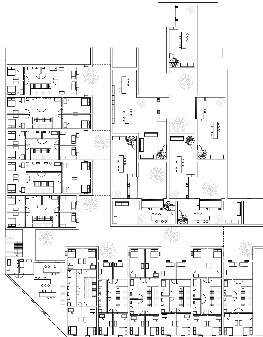
Grundriss 1 OG 1:200
