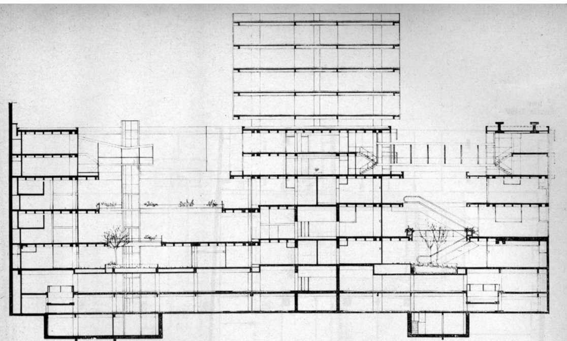
Corte transversal Escala 1:400
