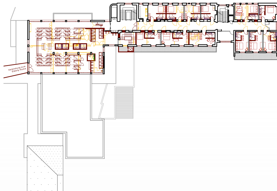
3. Obergeschoss - Garderobe des Hallenbads und Hotel Passarelle zu La Quercia
