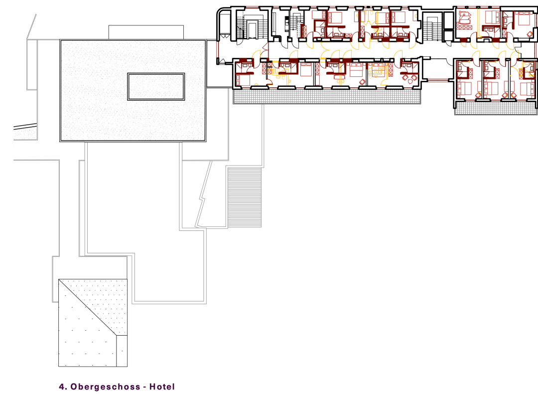
4. Obergeschoss - Hotel
