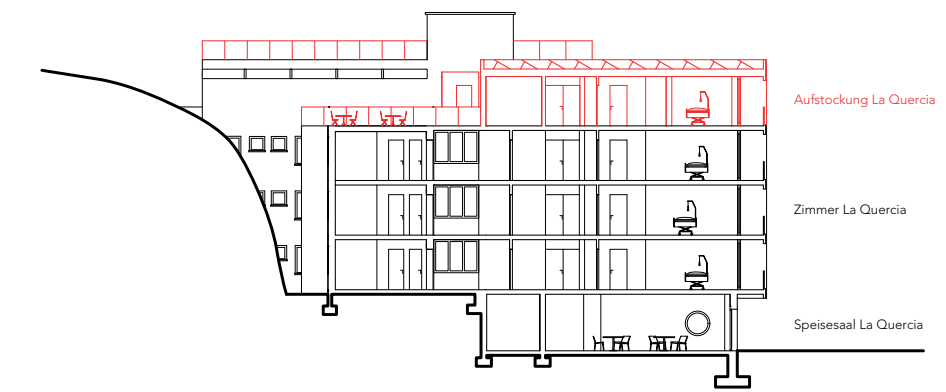
Querschnitt A-A 1:200
