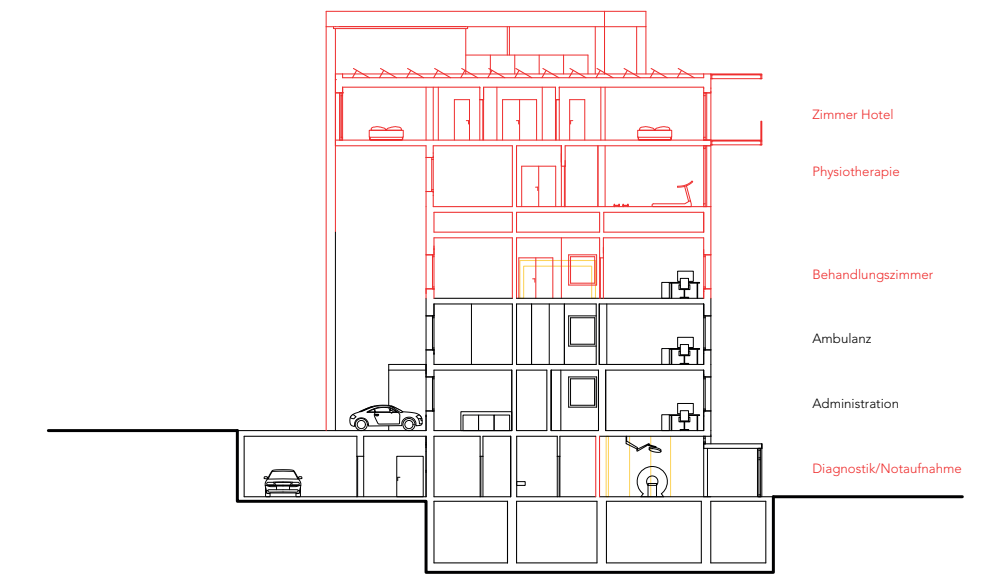
Querschnitt C-C 1:200
