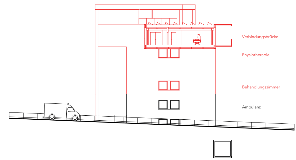
Querschnitt B-B 1:200
