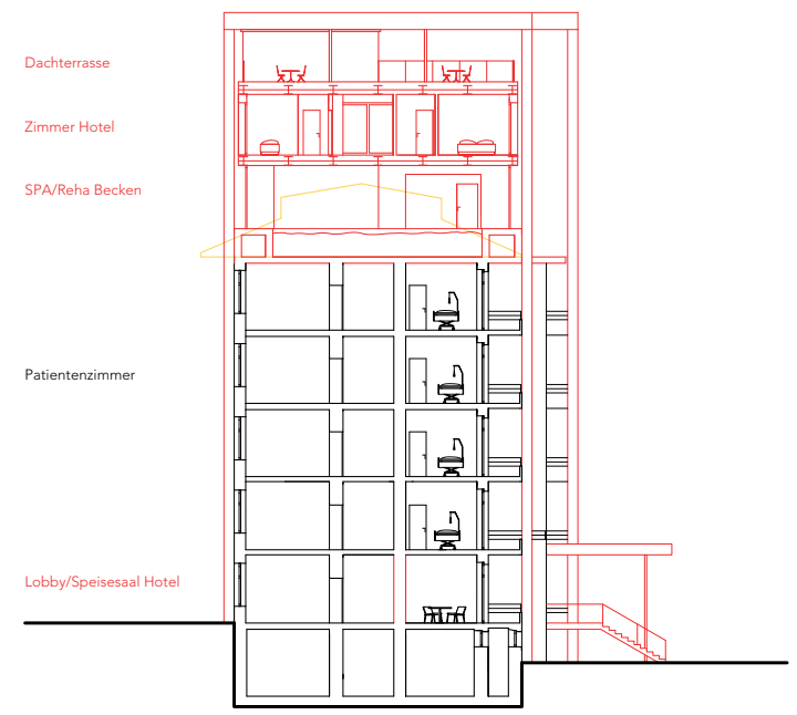
Querschnitt D-D 1:200
