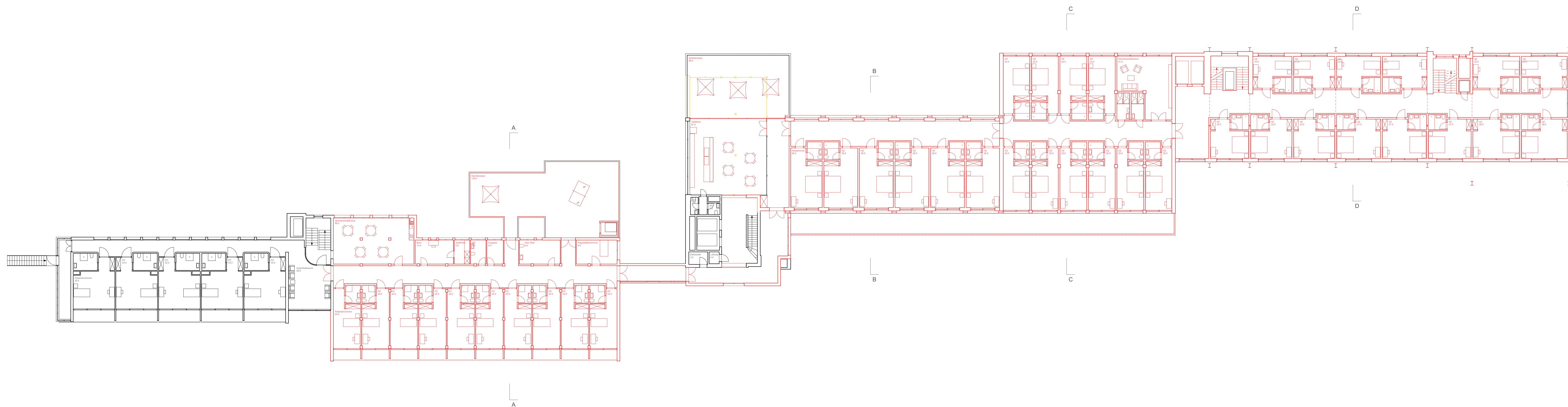
Grundriss 4. Obergeschoss 1:200
