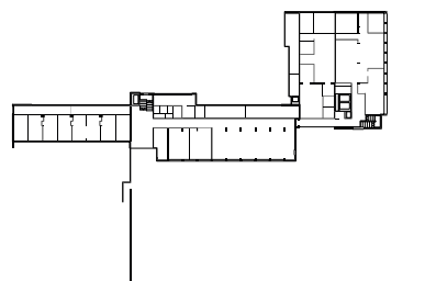
Grundriss 1, Obergeschoss 1:1000
