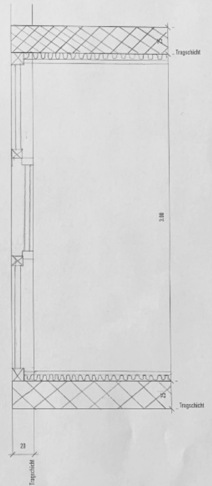
Schnitt 1:20
